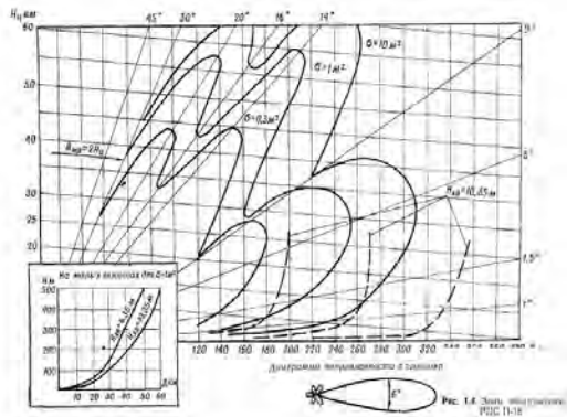
Рис. 1.3. Зоны обнаружения РЛС П-18.
